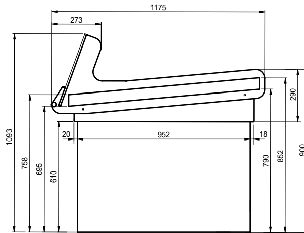
Vista laterale - BP 105 NV
