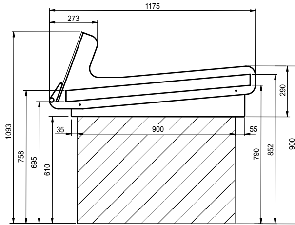
Vista laterale - VP 105 PV
