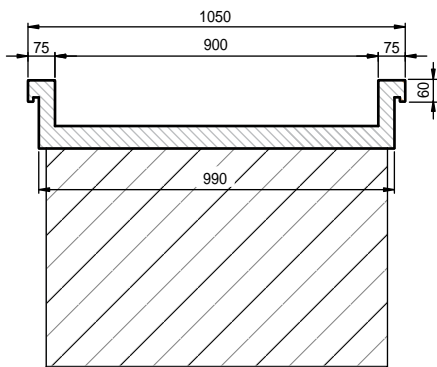
Vasca - Sez. A:A
