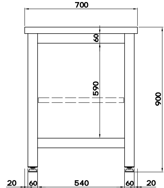
Sezione - Section A-A
